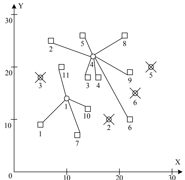
Рис. 3. Размещение базовых станций и абонентов после оптимизации
